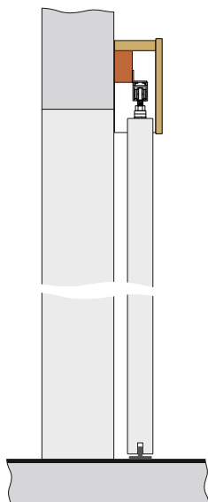
System naścienny zamontowany bez zabudowy
