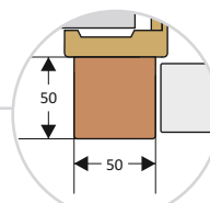
listwa odbojowa zamontowana na ościeżnicy
