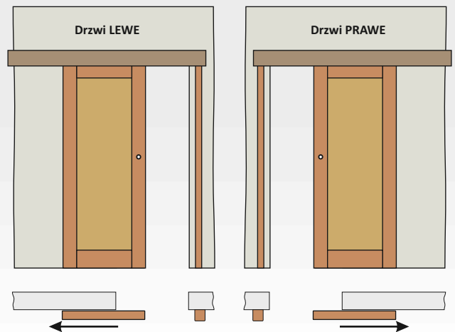
Wymiary szyn i maskownic:
