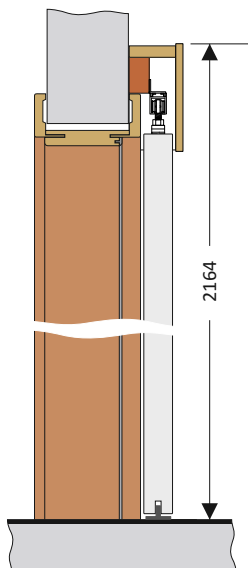
System naścienny zamontowany z zabudową tunelową
